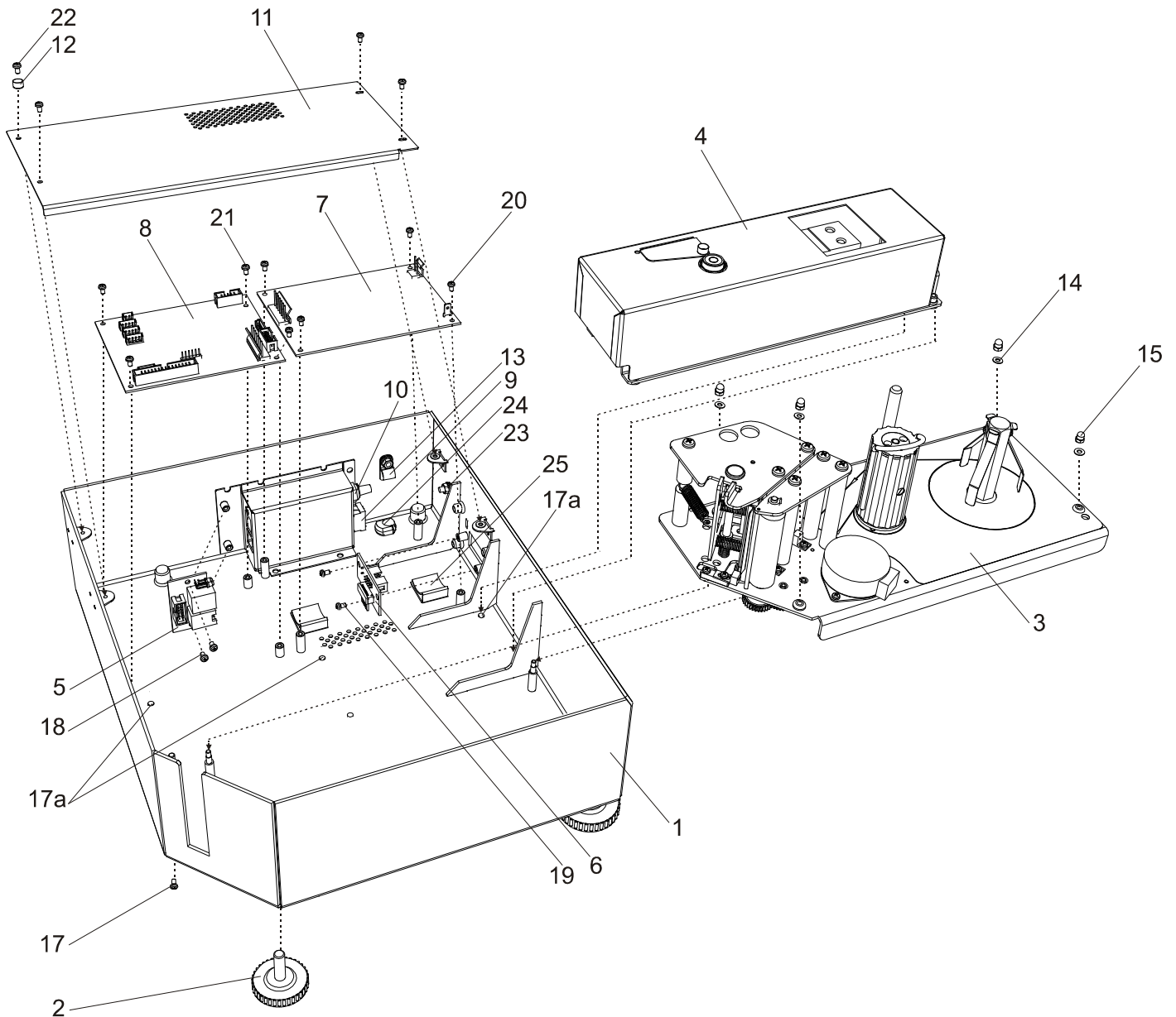
Рисунок 2. Весовой блок модели ШТРИХ-ПРИНТ 4.5
