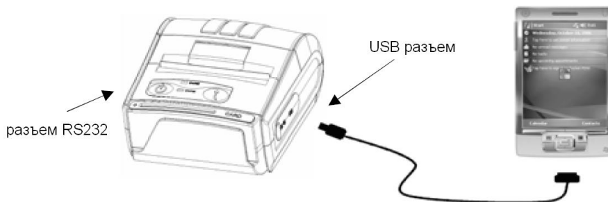
Рисунок 3 Подключение интерфейсного кабеля RS232/USB к ПК
